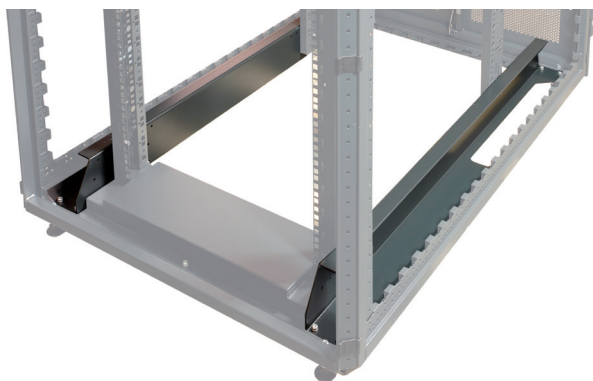
Высокая устойчивость и несущая способность 19" монтажного уровня
