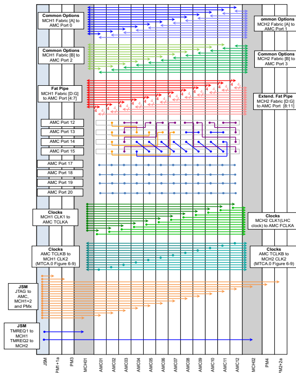
Топология объединительной платы
