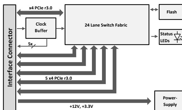
PCIe 24 Lane Switch Module Gen3
