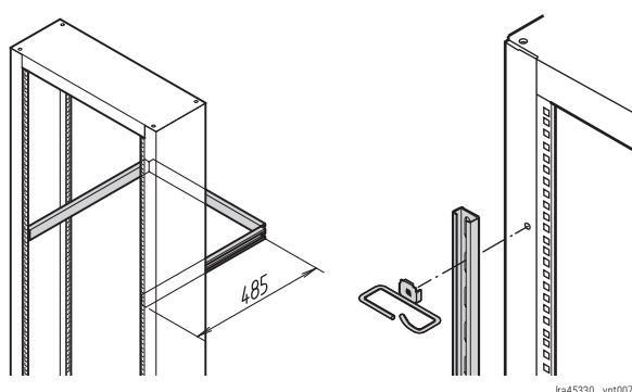
Организация укладки кабелей спереди и сзади
